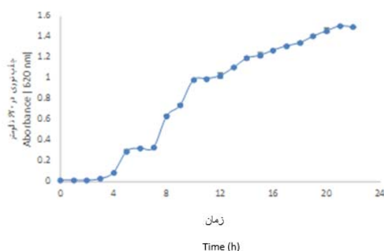
شکل ۱- منحنی رشد باکتری Pseudomonas putida Figure 1- Growth curve of Pseudomonas putida
