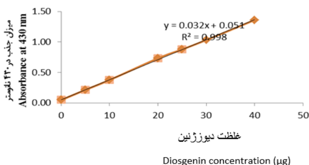
شکل ۳- نمودار استاندارد دیوزژنین Figure 3- Standard curve of diosgenin
